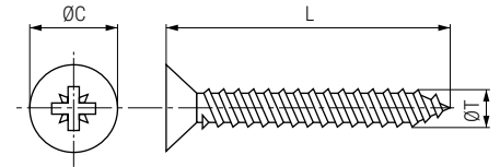
Pozidriv
