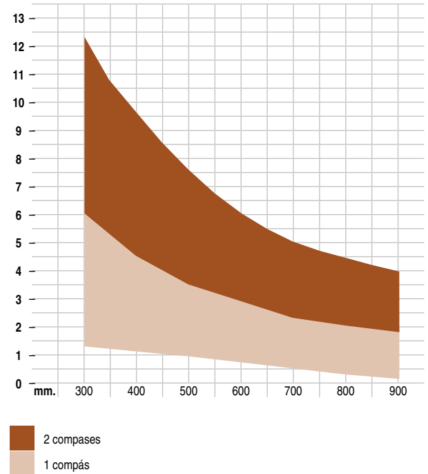
GRAFICO PARA ESTABLECER EL N.º DE COMPASES DE ACUERDO CON EL PESO DE LA PUERTA
