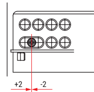
Presionar para enganchar el perno antivuelco.
