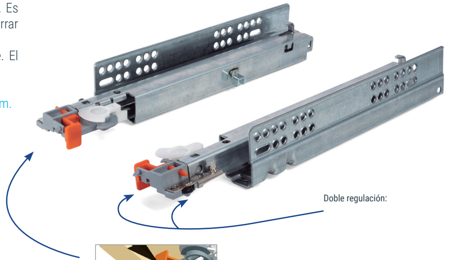
Presionar para enganchar el perno antivuelco.
