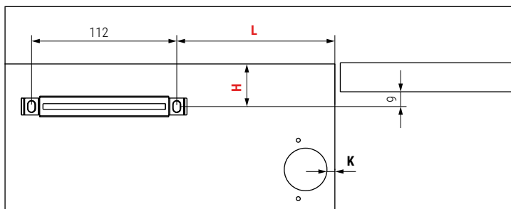
Colocación interna del mecanismo
